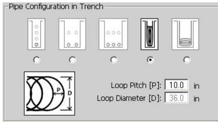
Fig. 5.4 Slinky Variables
